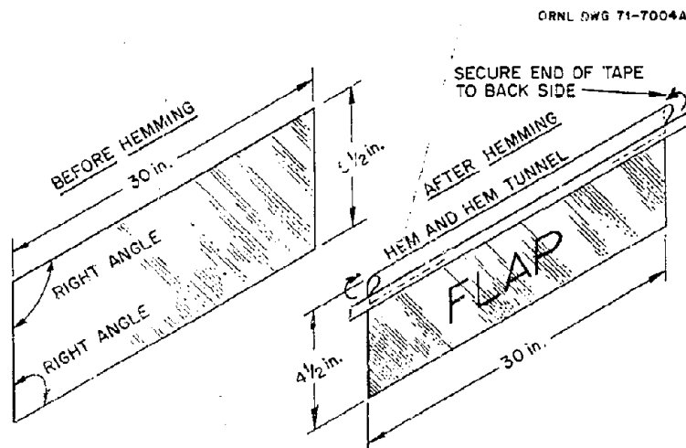
Fig. B-5. Flap pattern.
